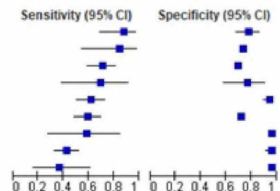
Зураг 4. Форест плот: PGI, PGR биомаркерын ходоодны хорт хавдрыг илрүүлэх чадамж
