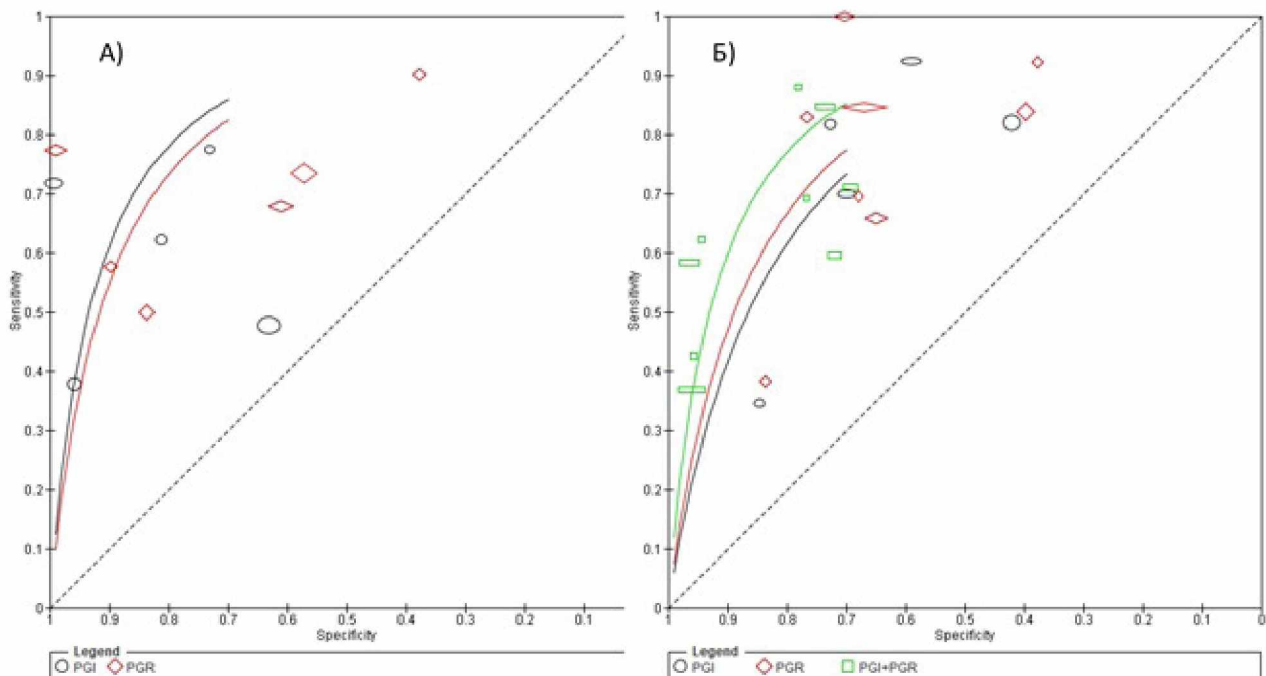
Зураг 5. Нэгтгэсэн ROC муруй.
